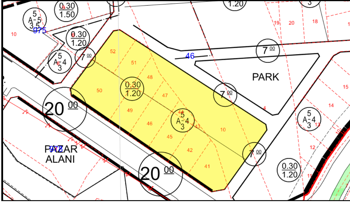
Şekil 4: 1/1000 Ölçekli Uygulama İmar Planı
